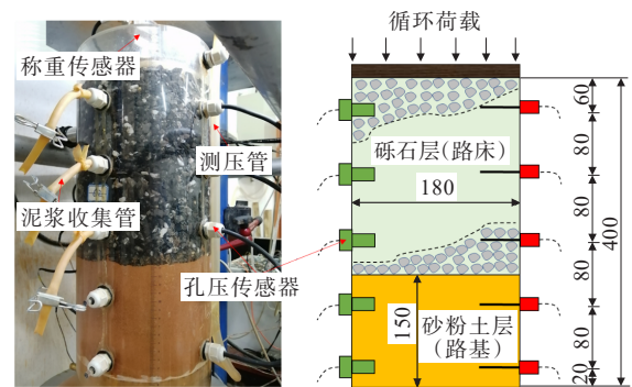
图2 加载前试样照片与结构示意图(单位:mm)
