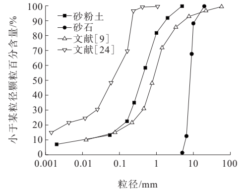
图1 试验材料的级配组成
