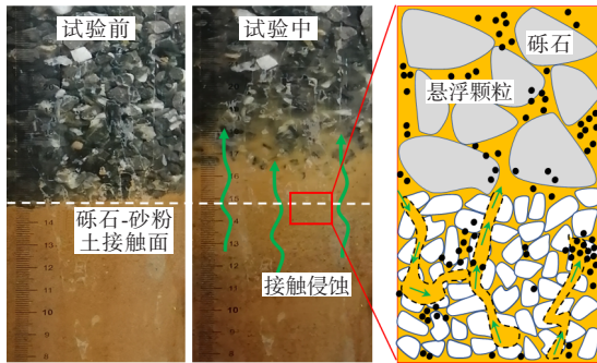
图5 抽吸效应诱发水-质迁移翻浆形成示意图
