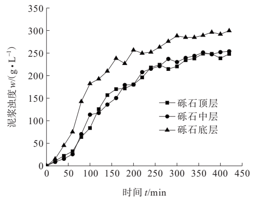
(a) 泥浆浊度
