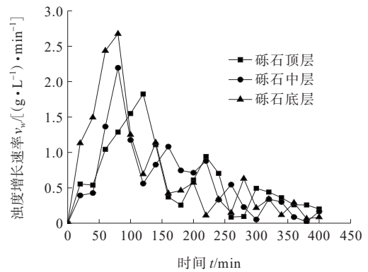
(b) 泥浆浊度增长速率
