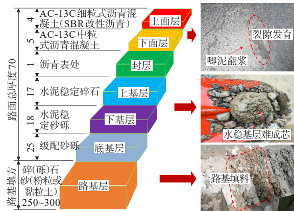
图8 G0615德马高速结构设计方案与病害取芯调查(单位:cm)
